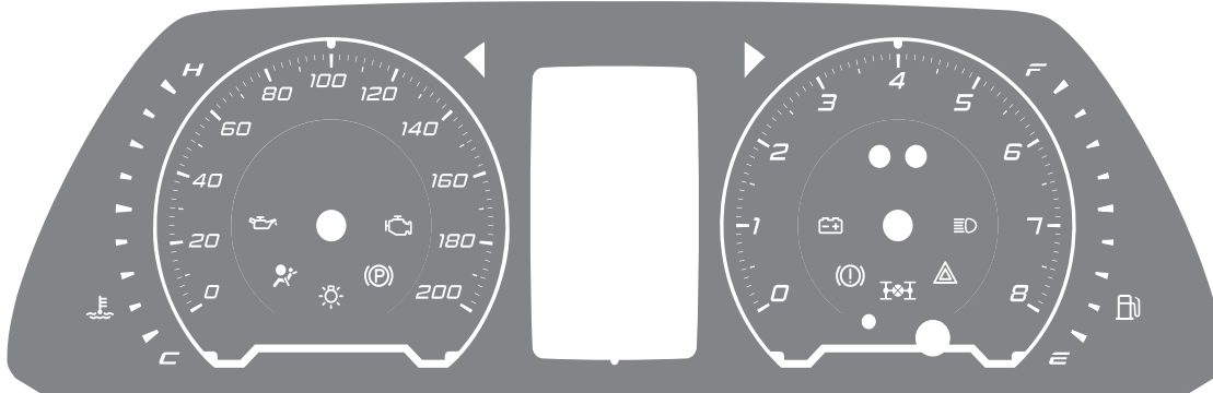
Рис. 14 Информационное поле ЭКП GF 825 CN.
