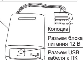
К-Line-адаптер (программатор) GF 911 производства «FERRUM»
